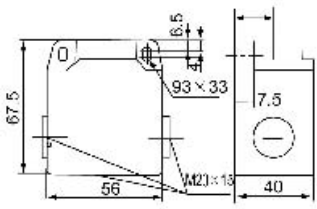
LXP1-100壳体尺寸
